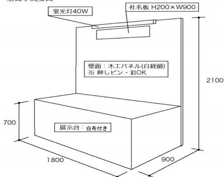
基礎小間姿図
